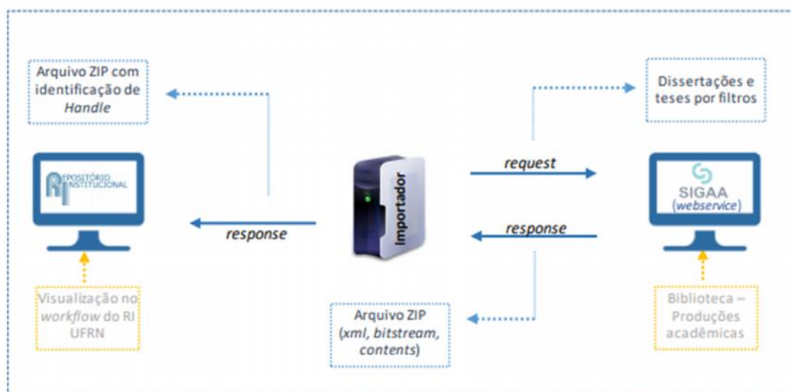
Figura 3 – Modelo de interoperabilidade entre SIGAA e RI UFRN
